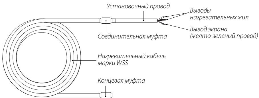
Конструкция кабеля нагревательного WSS
