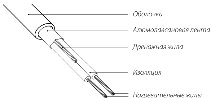
Конструкция кабеля нагревательного WSS
