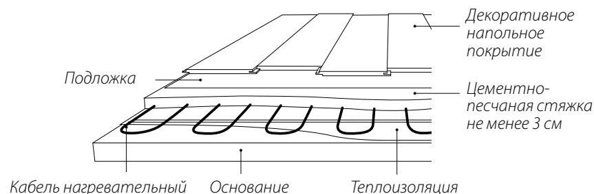
Схема укладки под ламинат, линолеум или ковролин
